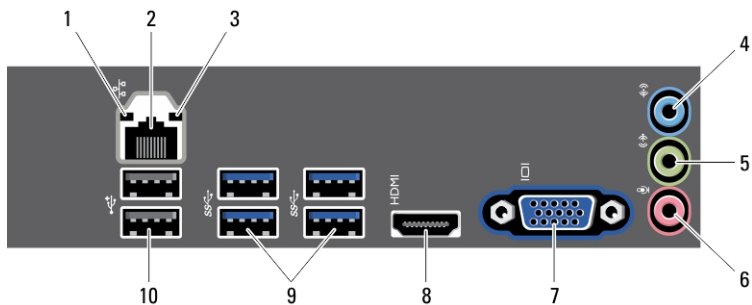
Ilustración 2. Vista del panel posterior
